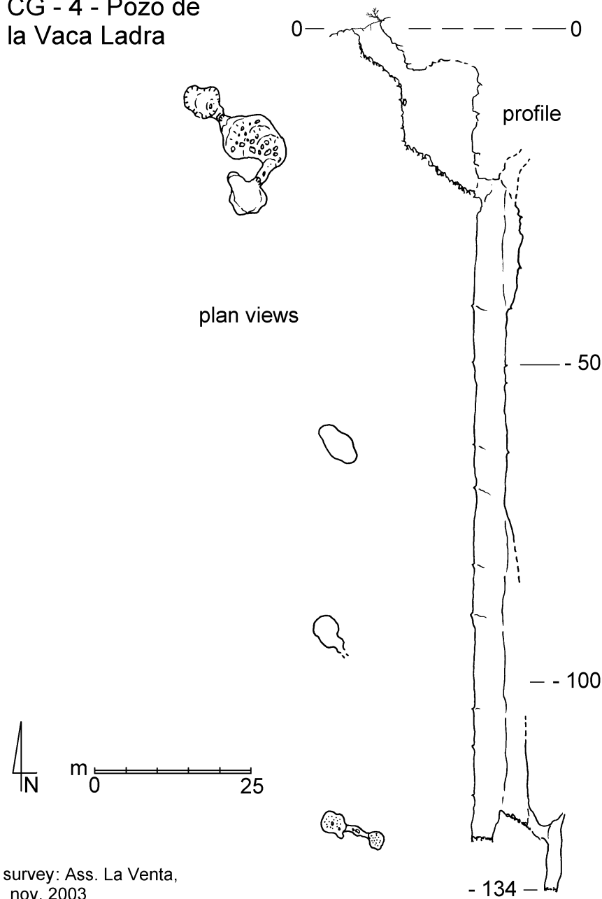
Fig. 10 - Plan views and longitudinal section of Pozo de la Vaca Ladra, Cerro Grande (survey: Ass. Geogr. La Venta).
